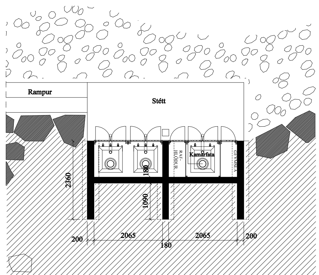
GRUNNMYND KJALLARI
