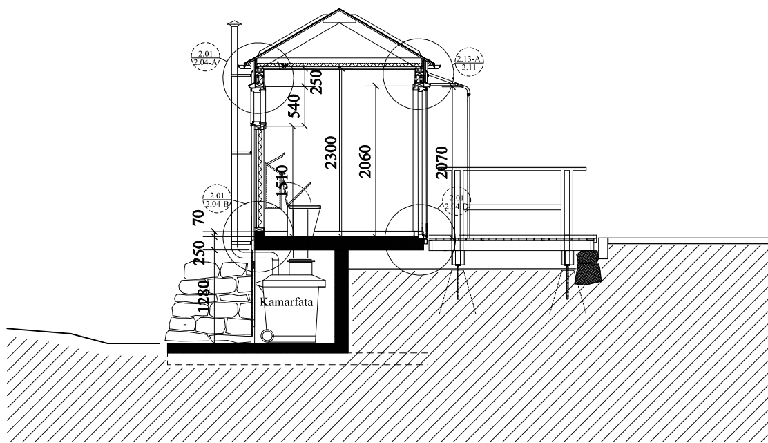
ÞVERSNEIÐING
